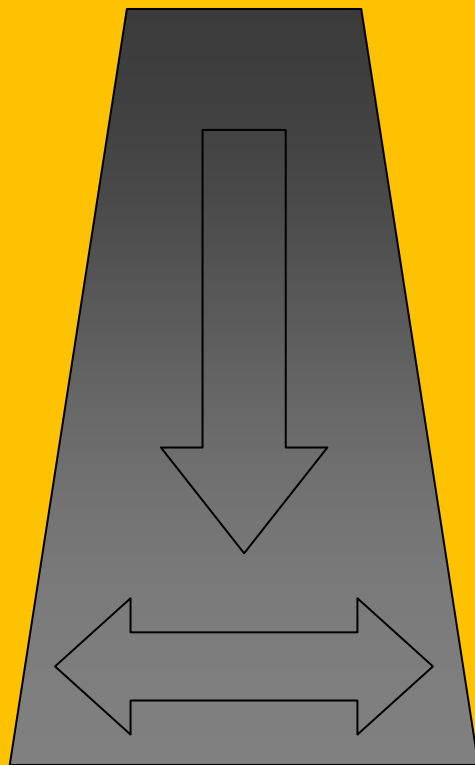
LÓGICA INCREMENTAL
